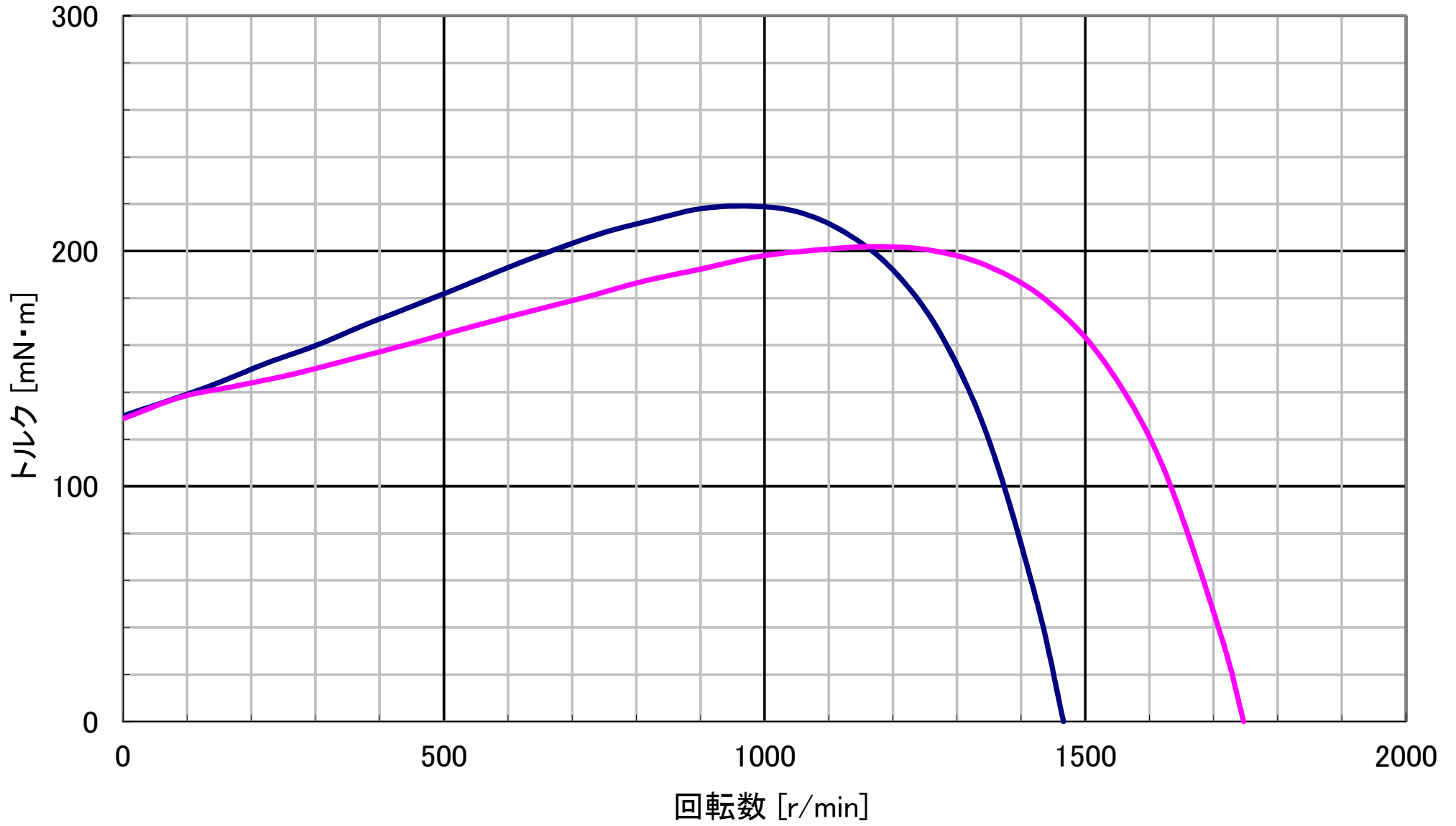
概略S-T特性(φ94シリーズ)
