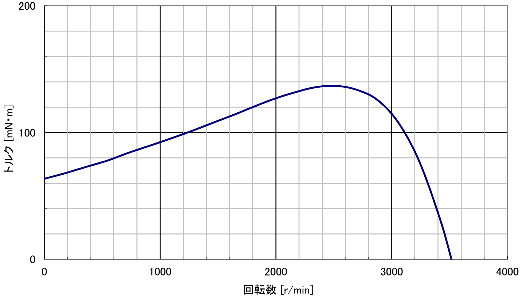
概略S-T特性(φ70シリーズ)
