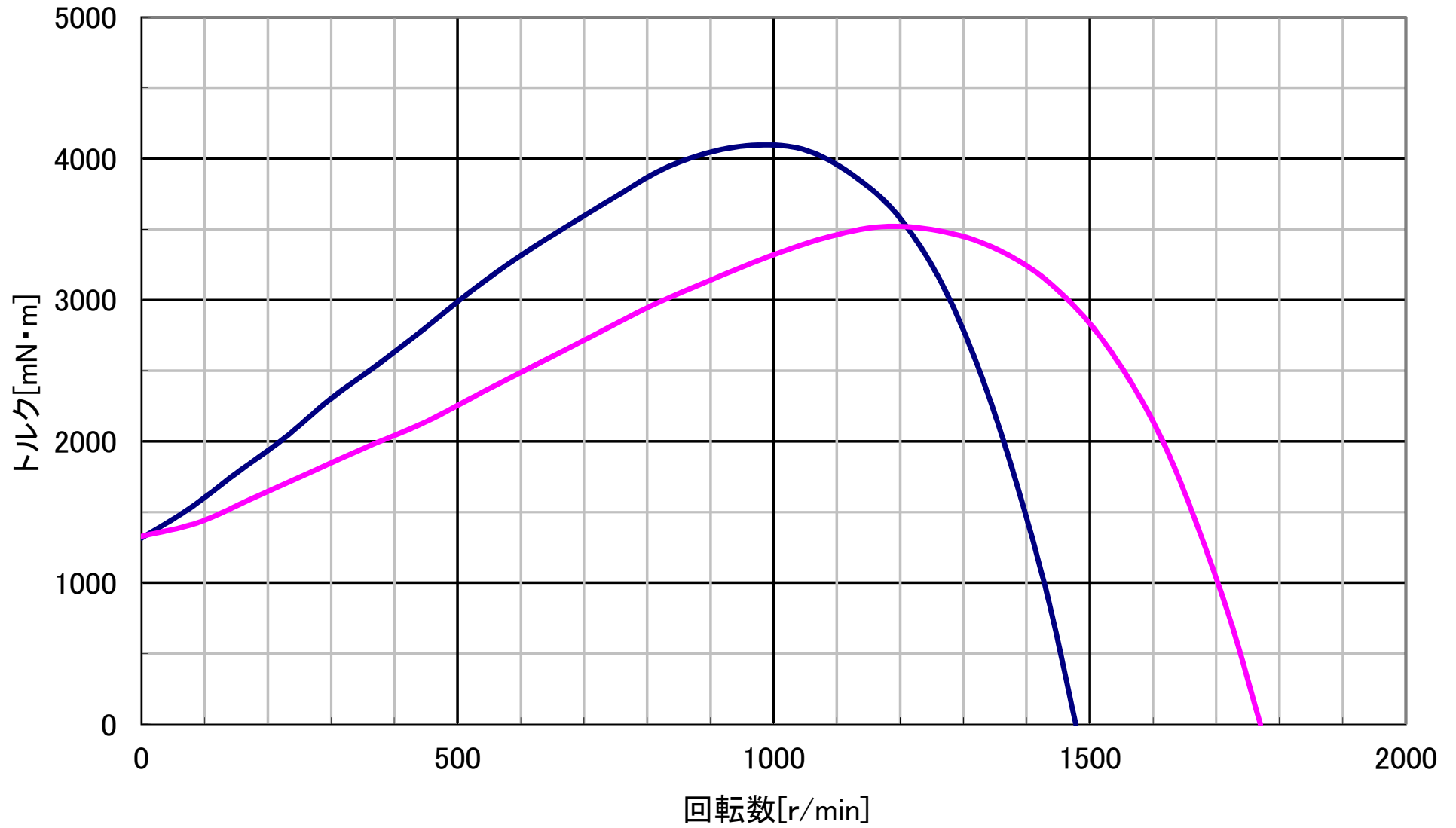
概略S-T特性(φ140シリーズ)
