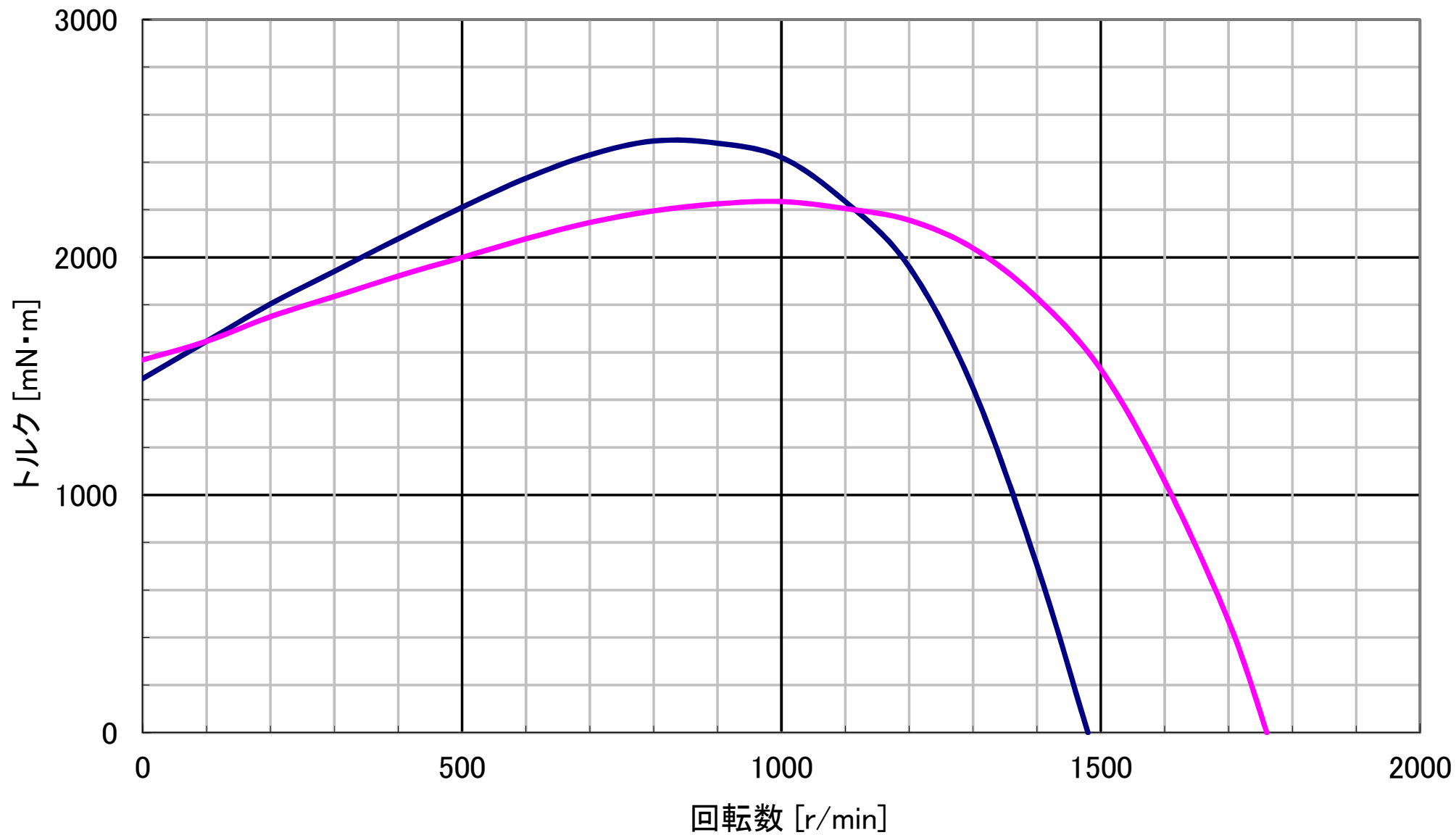
概略S-T特性(φ120シリーズ)
